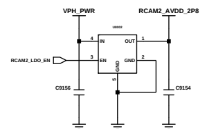
RCAM2_AVDD
